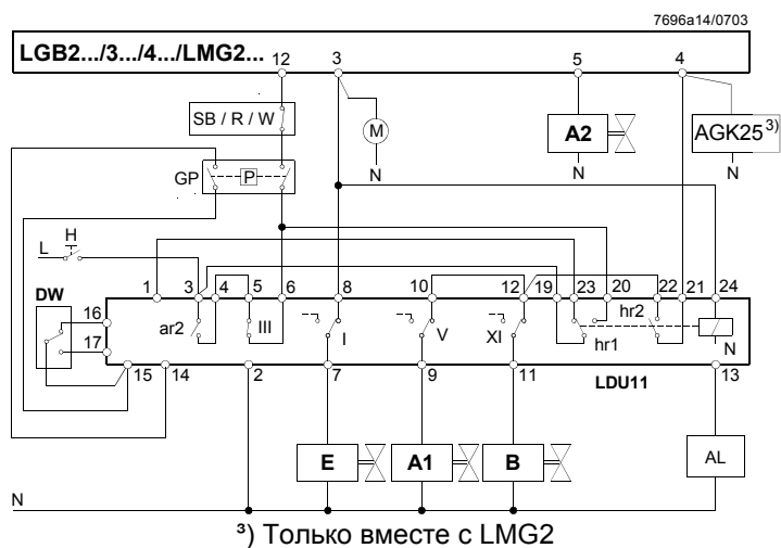
Установки без трубы сброса в атмосферу
