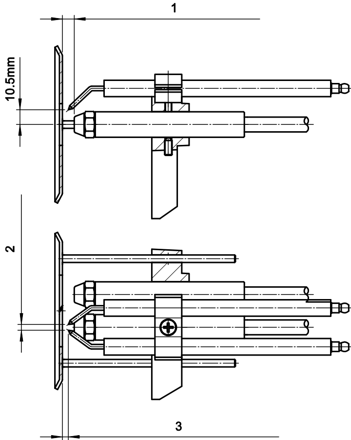
Fig. 13 УСТАНОВКА ЭЛЕКТРОДОВ
