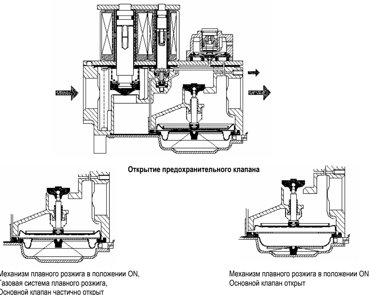
Рис. 16. Модели плавного розжига с сервоприводом.
