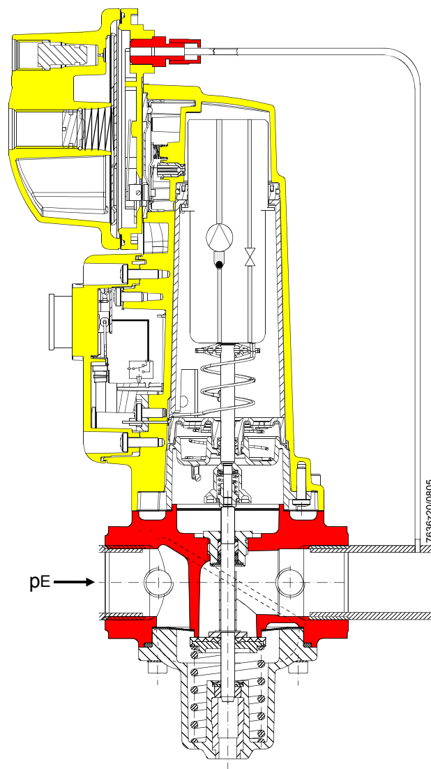
Разрез VGG... с приводом SKP25...
