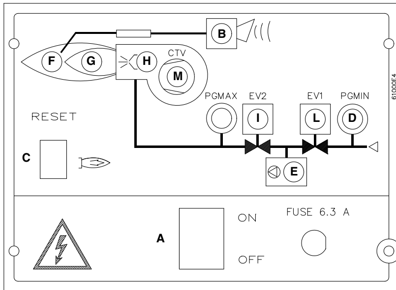
Рис. 25 - Передняя панель электроцита
