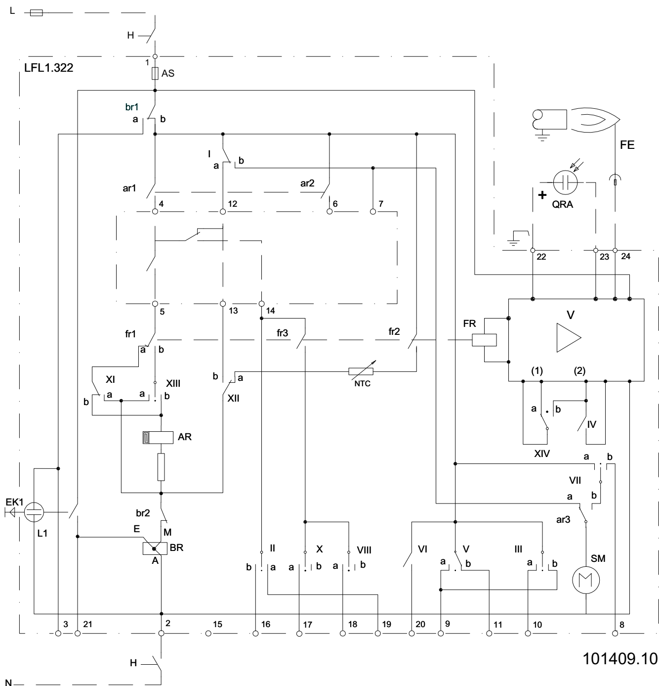
Схема LFL 1.322
