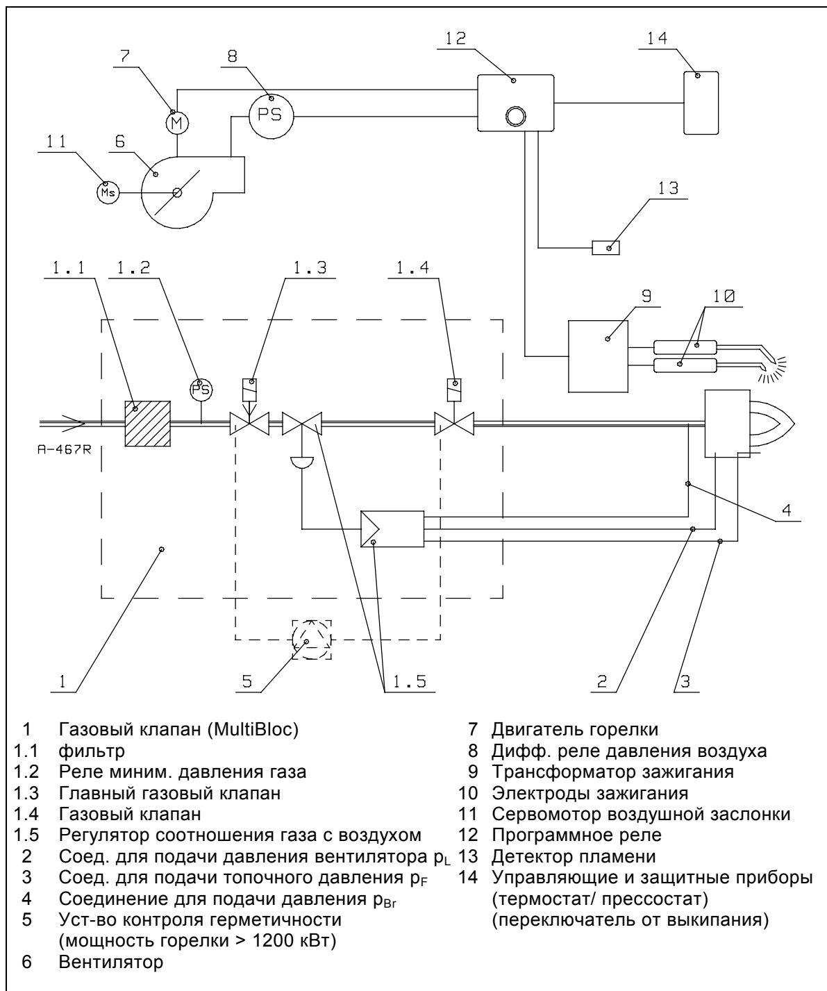
Схема № A-467R
