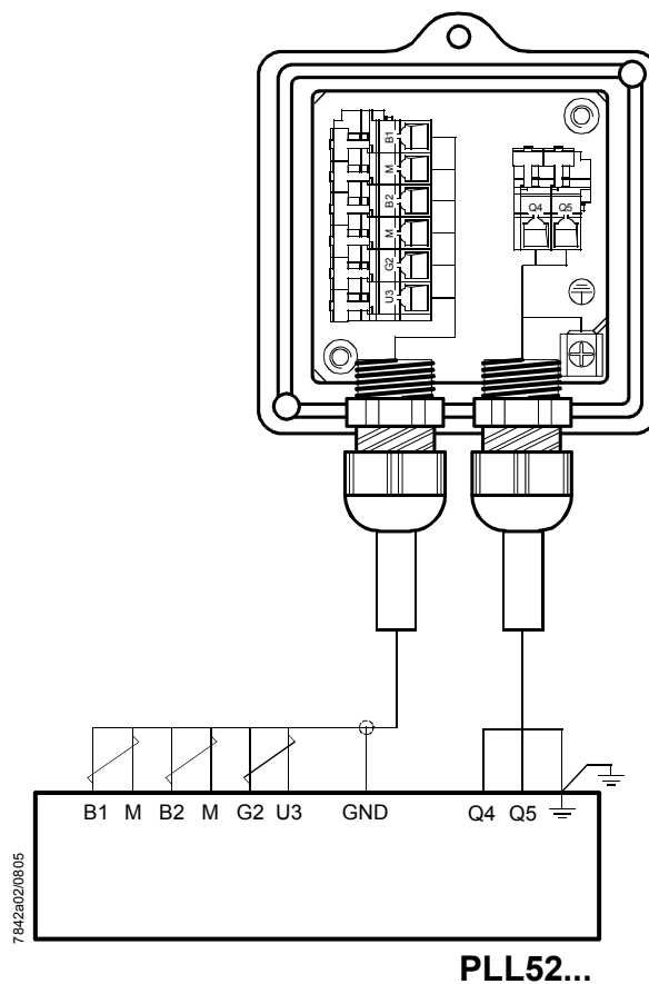
Рис.8: Электрическое подключение
